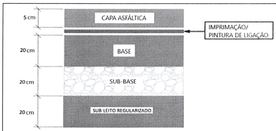
Figura 21 - Serviço 1: Pavimento novo com aplicação de CBUQ
